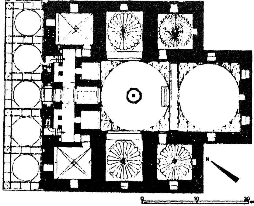
الشكل ٢٢-١٢ خطة جامع يشيل ( بنية الوحدات المقبية ) بورصة، تركيا ١٤١٢-١٤١٩ م.
